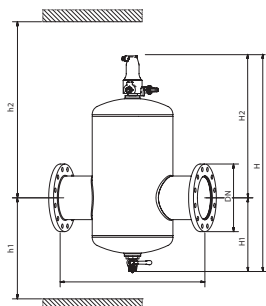
Сепараторы микропузырьков
