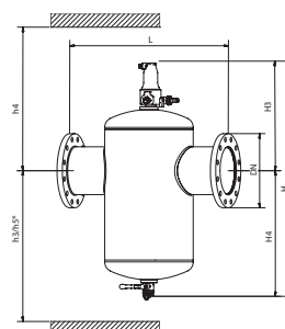
Сепараторы шлама
