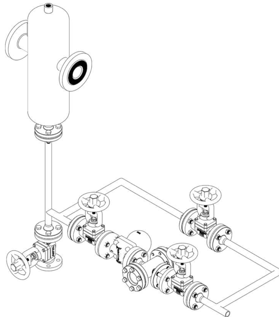
Узел отвода конденсата УОК в комплектации с поплачковым конденсатоотводчиком, байпасной линией и сепаратором пара
