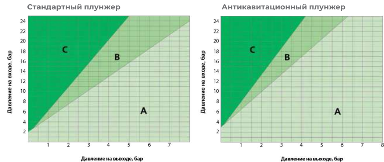
Кавитационный график
