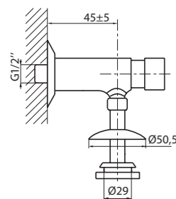
Кран для писсуара с наружной подводкой 8420 90 0
