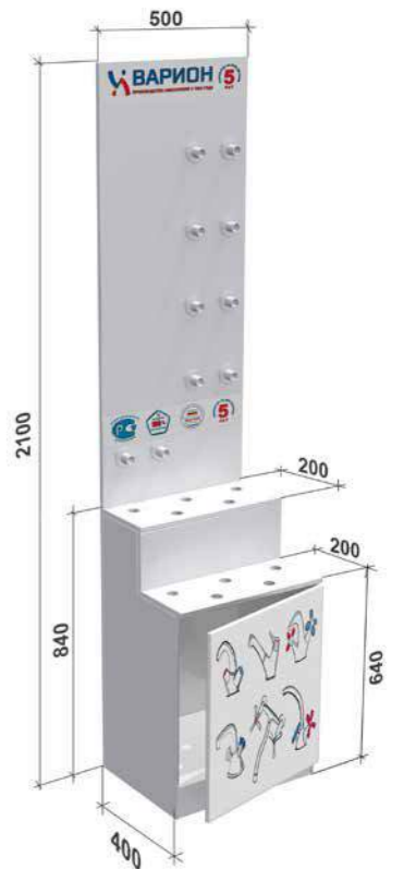
5990 39 0 Стенд для смесителей и душевых стоек узкий
