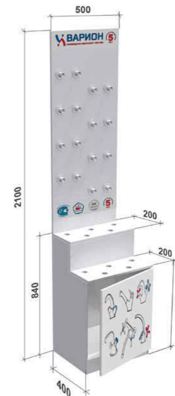
5990 35 0 Стенд для смесителей узкий
